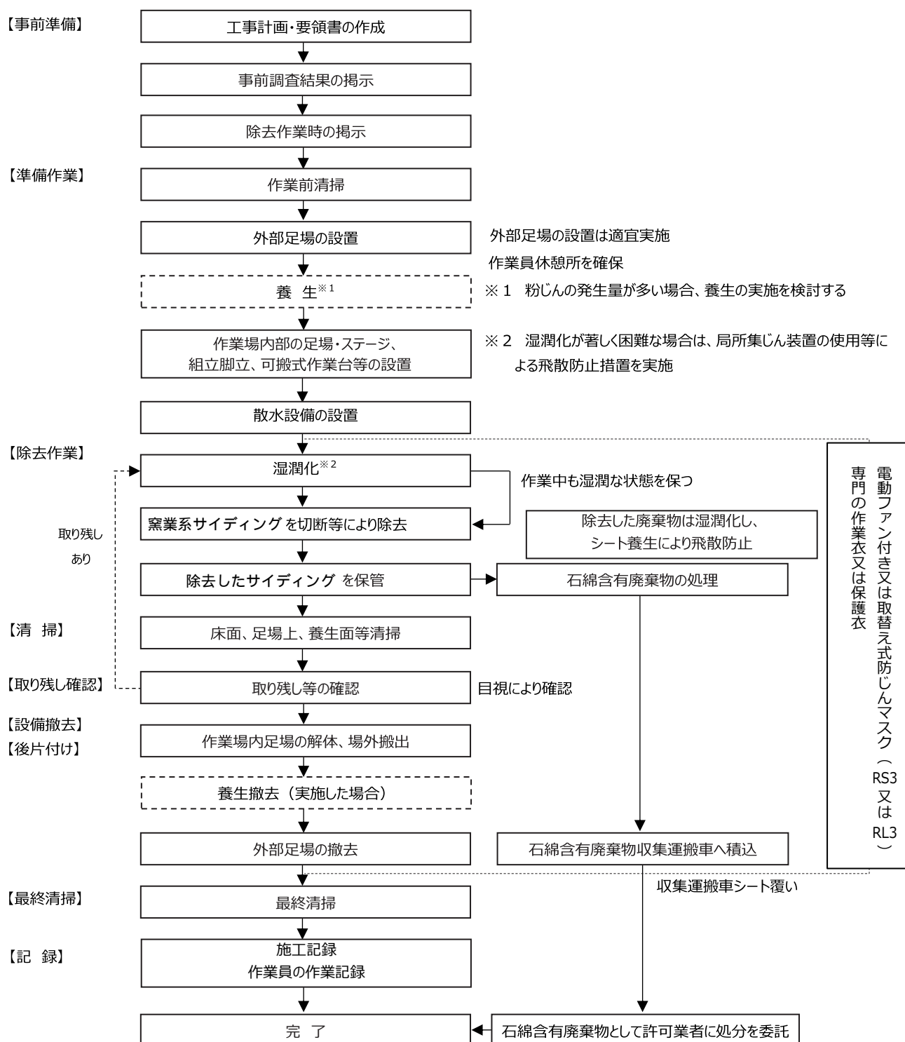
図 石綿含有窯業系サイディングを切断等により除去する場合の作業手順
